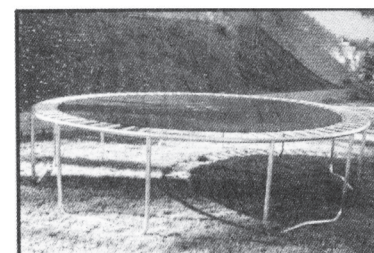
4. Upevněte zbývající pružiny. Dodržujte vždy protilehlé upevňování pružin, aby nedošlo k jejich poškození!
